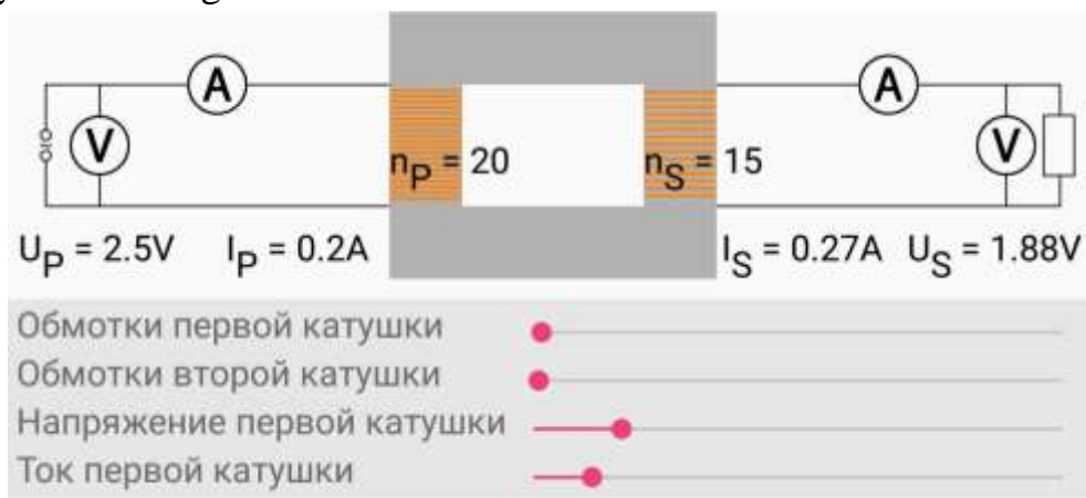
Transformatorning ishlash prinsipi
