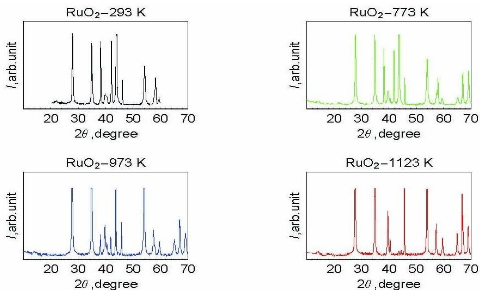
7a-rasm. Erkin RuO 2 ning rengenogrammalari
